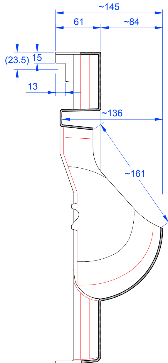
Schnitt B-B
